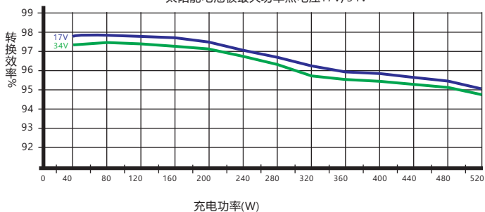
12V系统转换效率曲线 太阳能电池板最大功率点电压17V/34V
