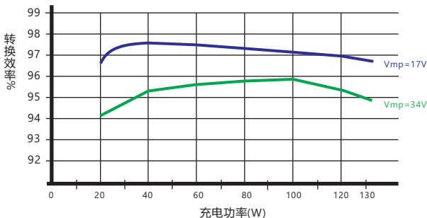
12V系统转换效率曲线 太阳能电池板最大功率点电压17V
