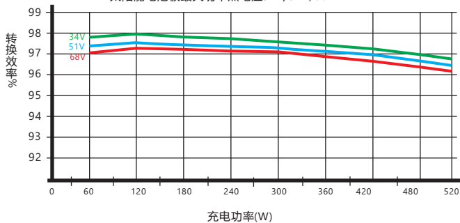
24V系统转换效率曲线 太阳能电池板最大功率点电压34V/51V/68V
