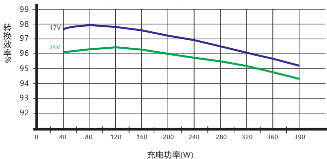
12V系统转换效率曲线 太阳能电池板最大功率点电压17V/34V
