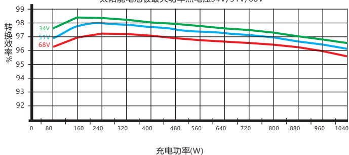
24V系统转换效率曲线 太阳能电池板最大功率点电压34V/51V/68V
