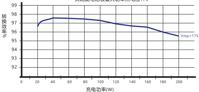
12V系统转换效率曲线 太阳能电池板最大功率点电压17V
