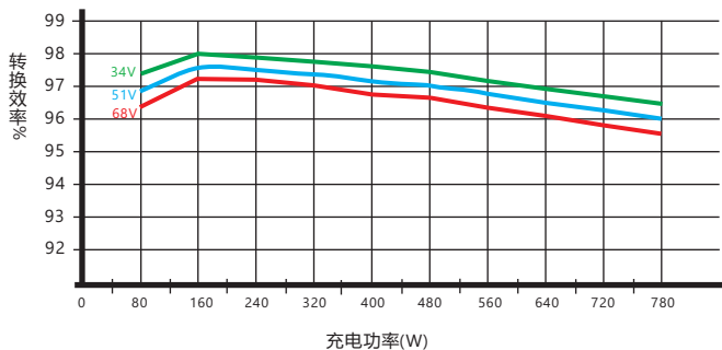
24V系统转换效率曲线 太阳能电池板最大功率点电压34V/51V/68V
